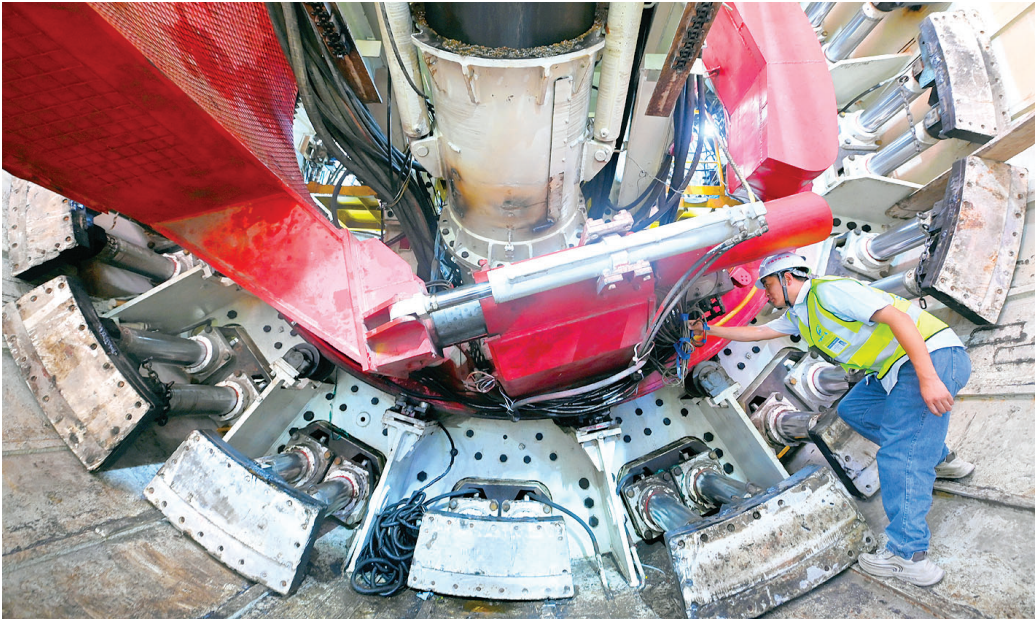
5月26日,施工人员在“青年先锋号”盾构机始发前检查设备。当日,由中铁一局承建的天津轨道交通Z4线6标段“青年先锋号”盾构机顺利始发,标志着Z4线关键区间隧道建设进入攻坚阶段。
