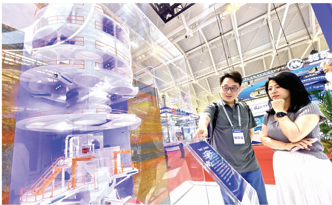
世界首台超大直径全断面硬岩竖向掘进机(模型)亮相展会。
