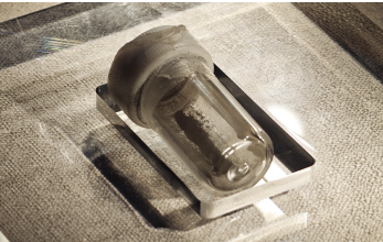
嫦娥六号带回的月球背面样品
