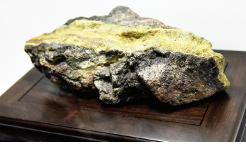
铀矿石标本——“开业之石”
